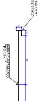
CORTE - A-A
